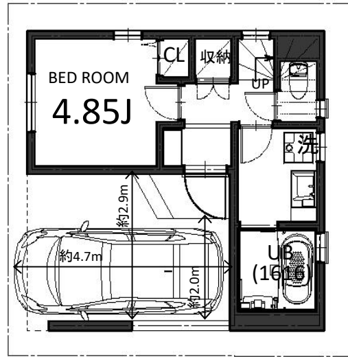
1F : 35.71 m 2 (車庫面積10.35㎡含む)
